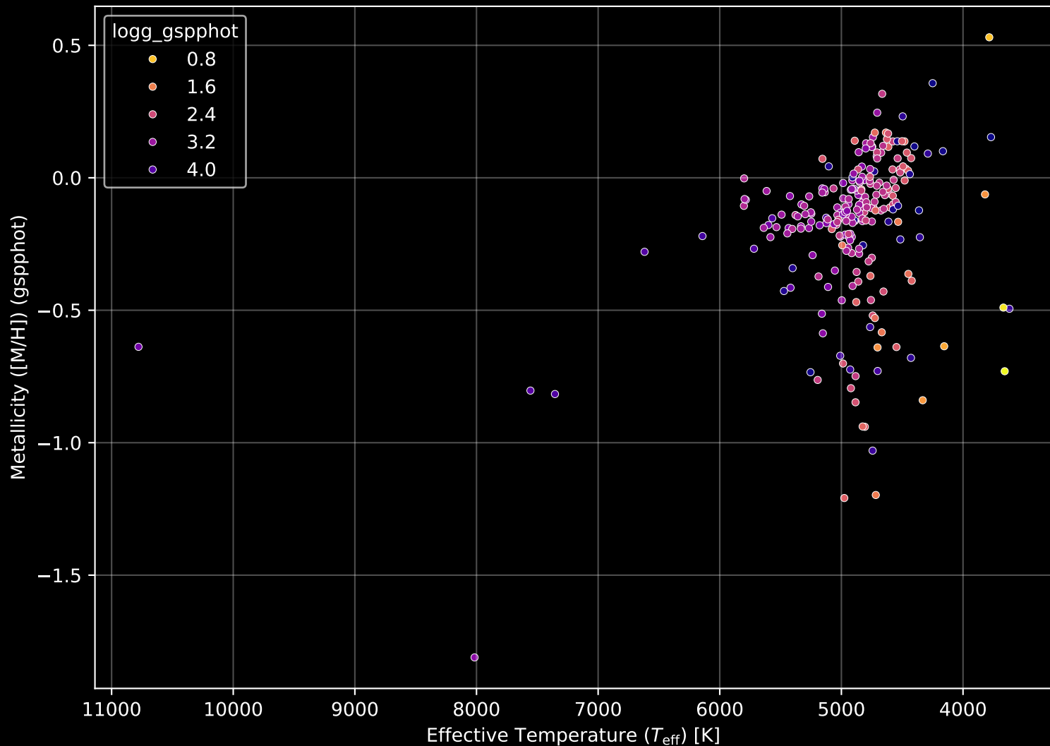
APOGEE DR17 Field: [296-12] Stellar Population Parameters (n= 239)
